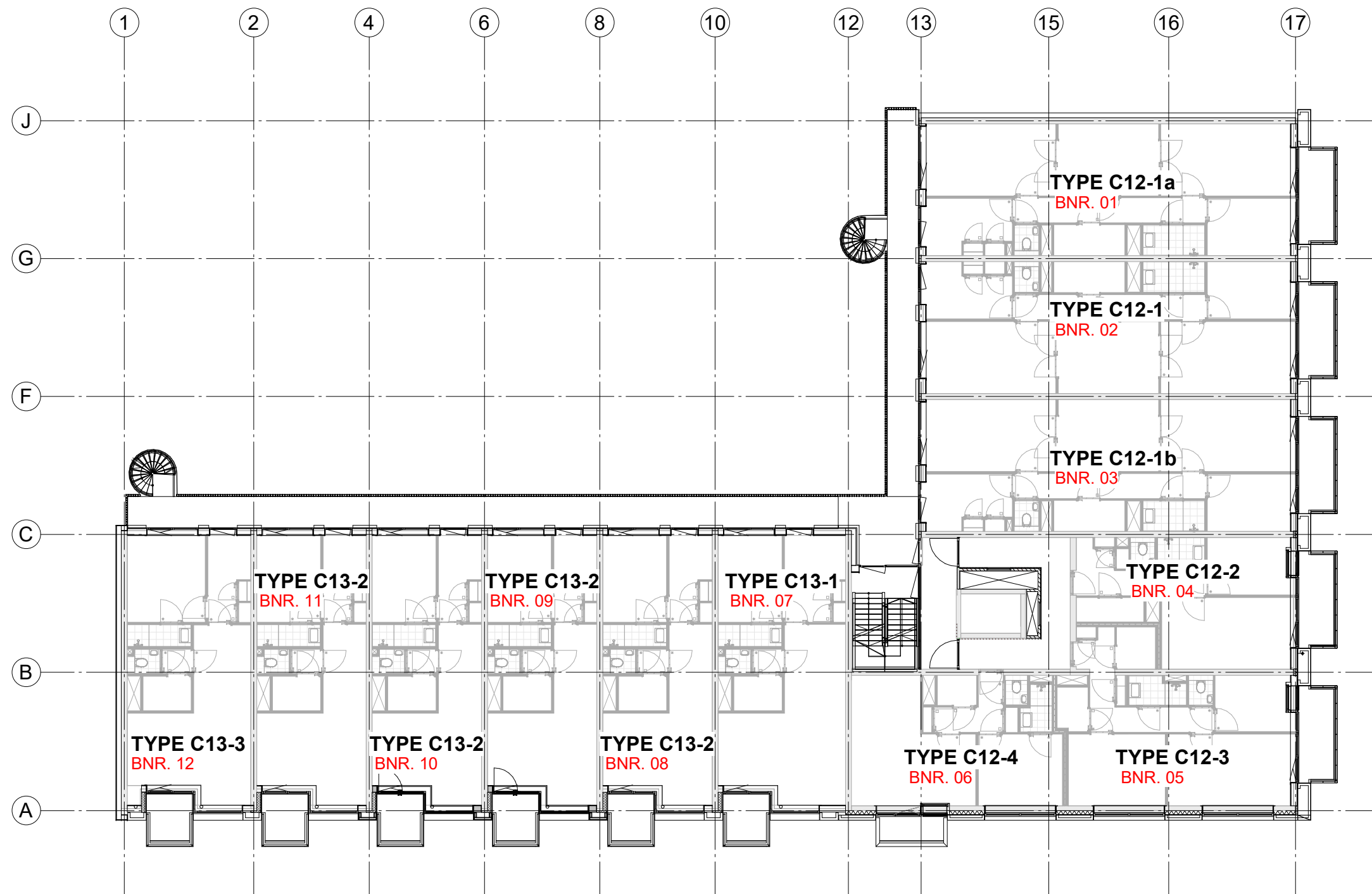
1E VERDIEPING
