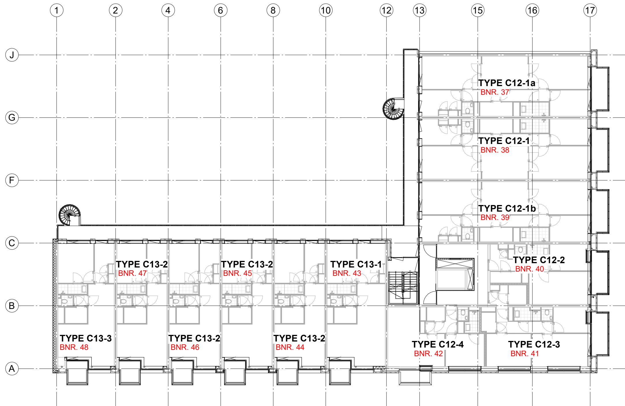
4E VERDIEPING
