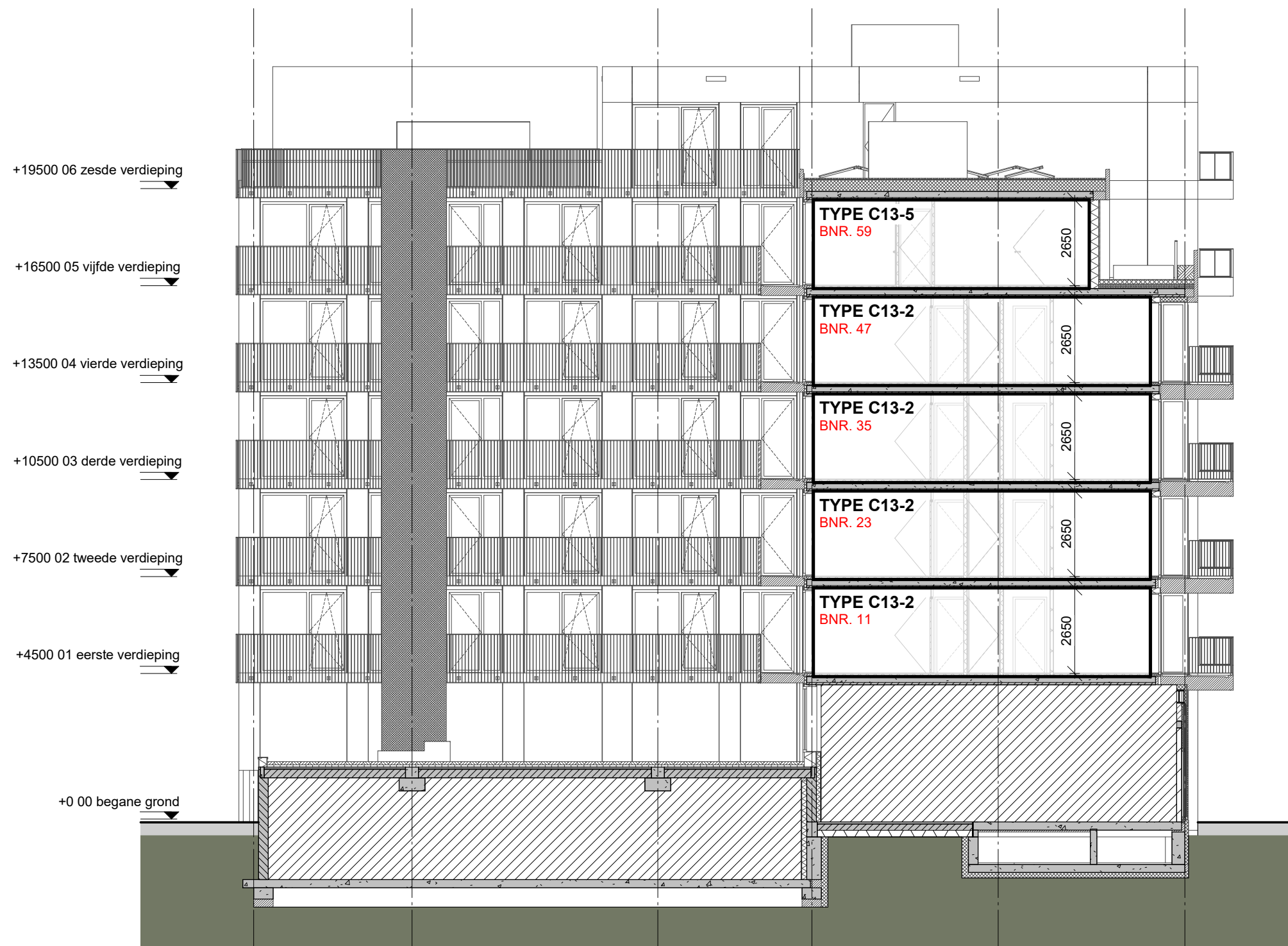
DOORSNEDE B-B
