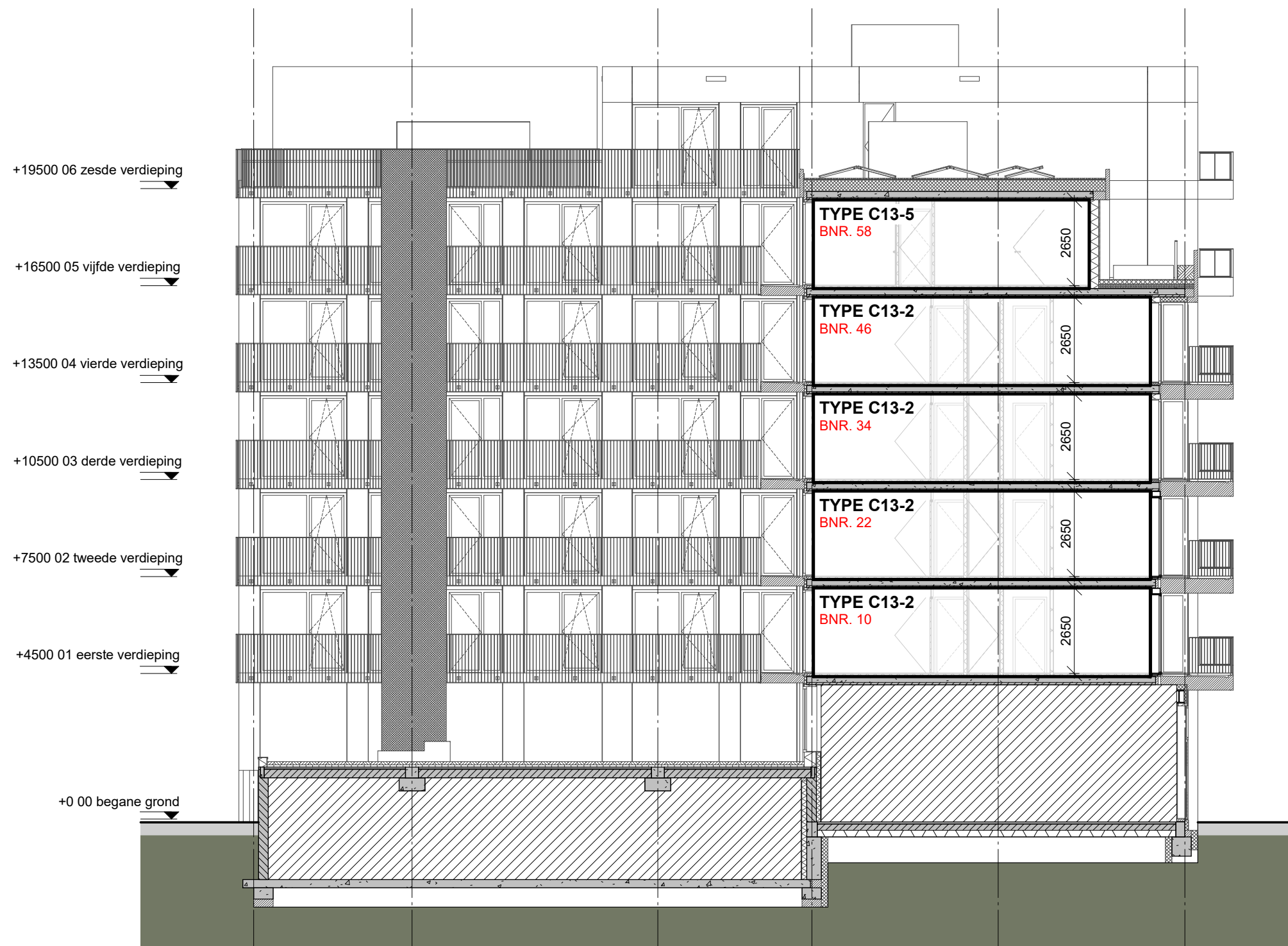
DOORSNEDE C-C
