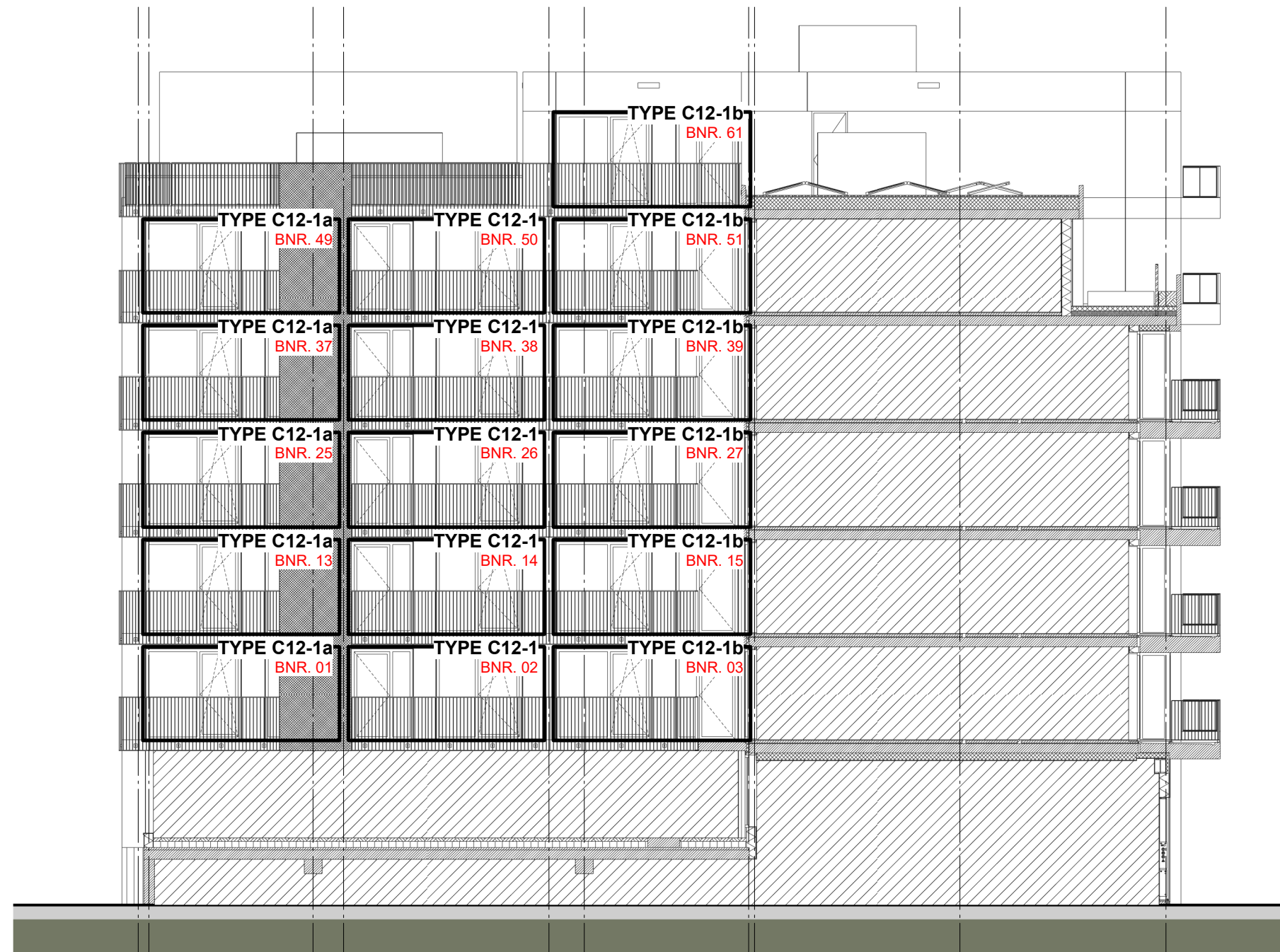
BINNENGEVEL VUURWERKERWEG
