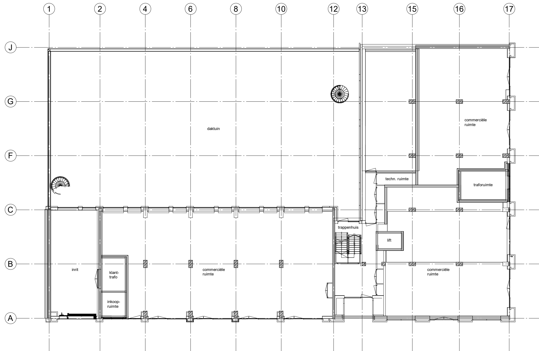
BEGANE GROND
