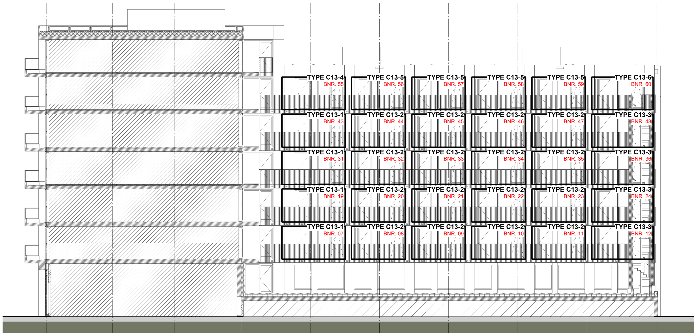
BINNENGEVEL SLIJPERWEG
