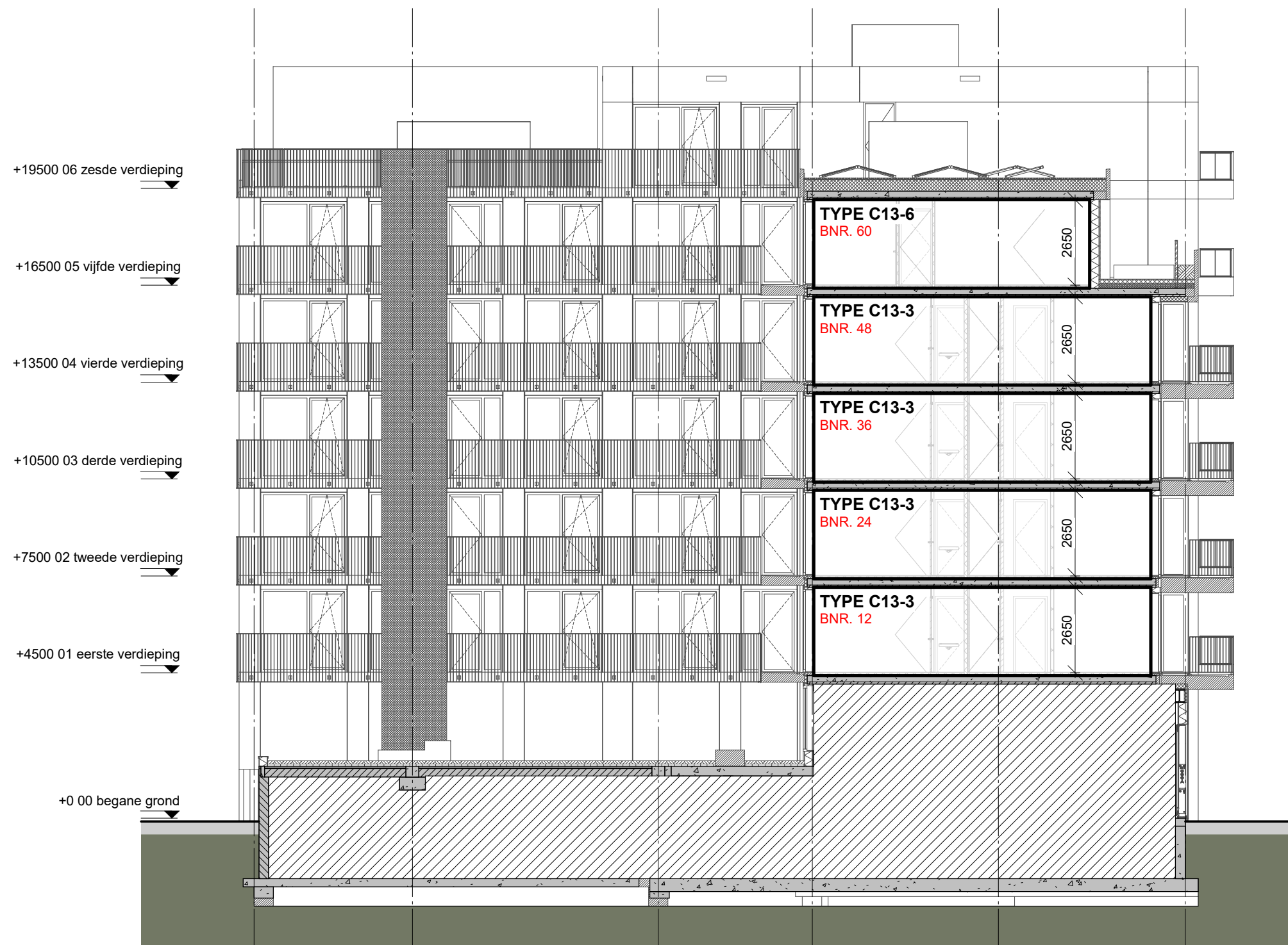
DOORSNEDE A-A
