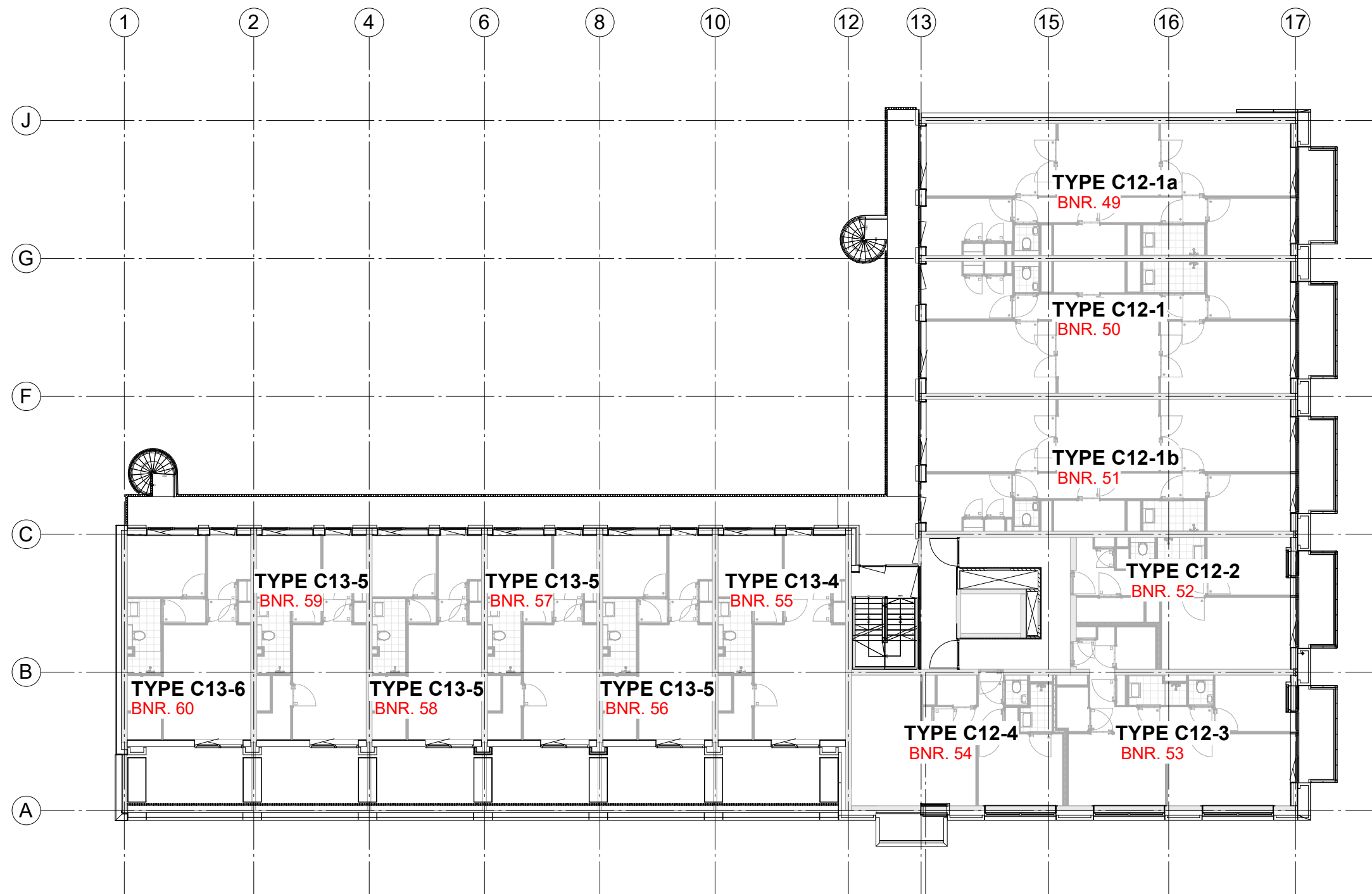
5E VERDIEPING
