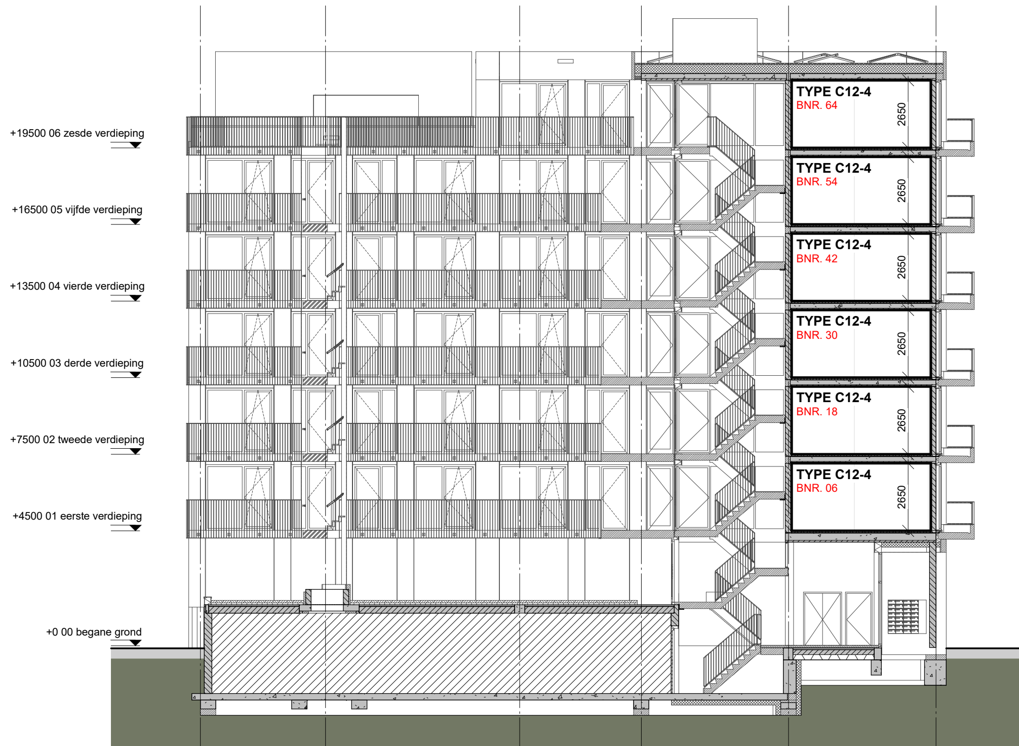
DOORSNEDE D-D
