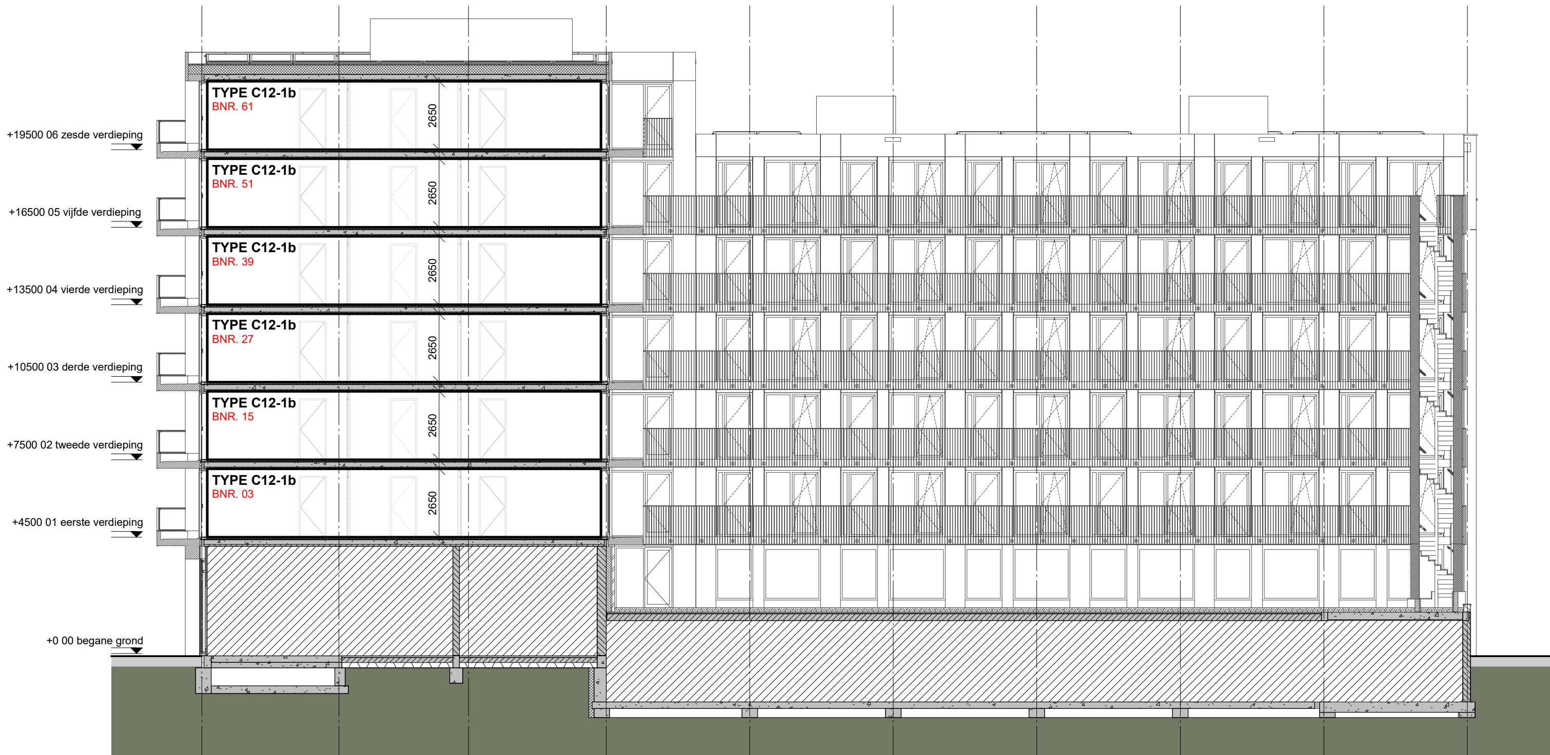
DOORSNEDE F-F
